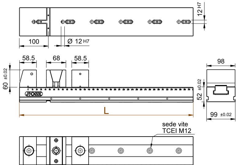
Morsa multipresa taglia 100 completo di n° 1 presa pezzo TIPO "CW" (2x1) corsa 2mm+2mm
